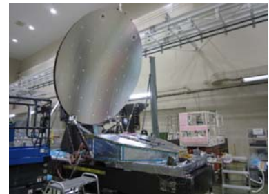
図15: CPR エンジニアリングモデル組立状況
