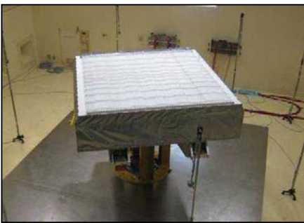
全球降水観測衛星/二周波降水レーダ (GPM/DPR)の音響試験 (平成21年3月)
