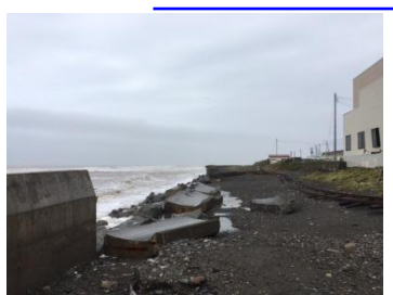
【護岸倒壊】 日高線 新冠～静内 80k328m付近
