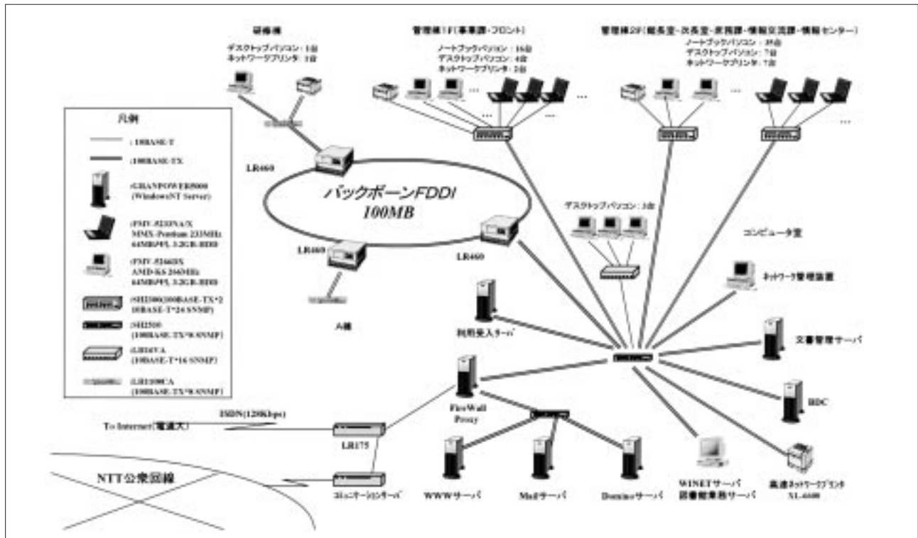
〈図1〉 国立婦人教育会館システム構成図
