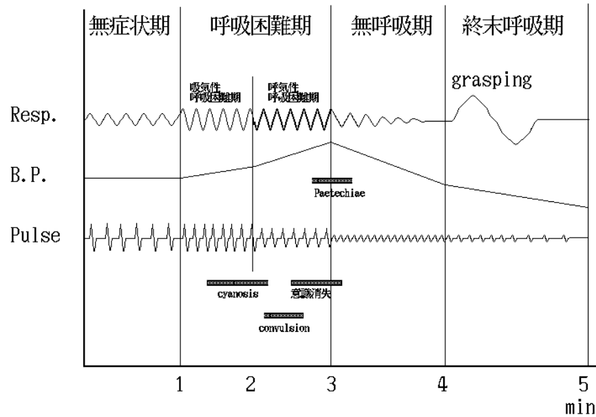
図 10.1: 窒息の経過
