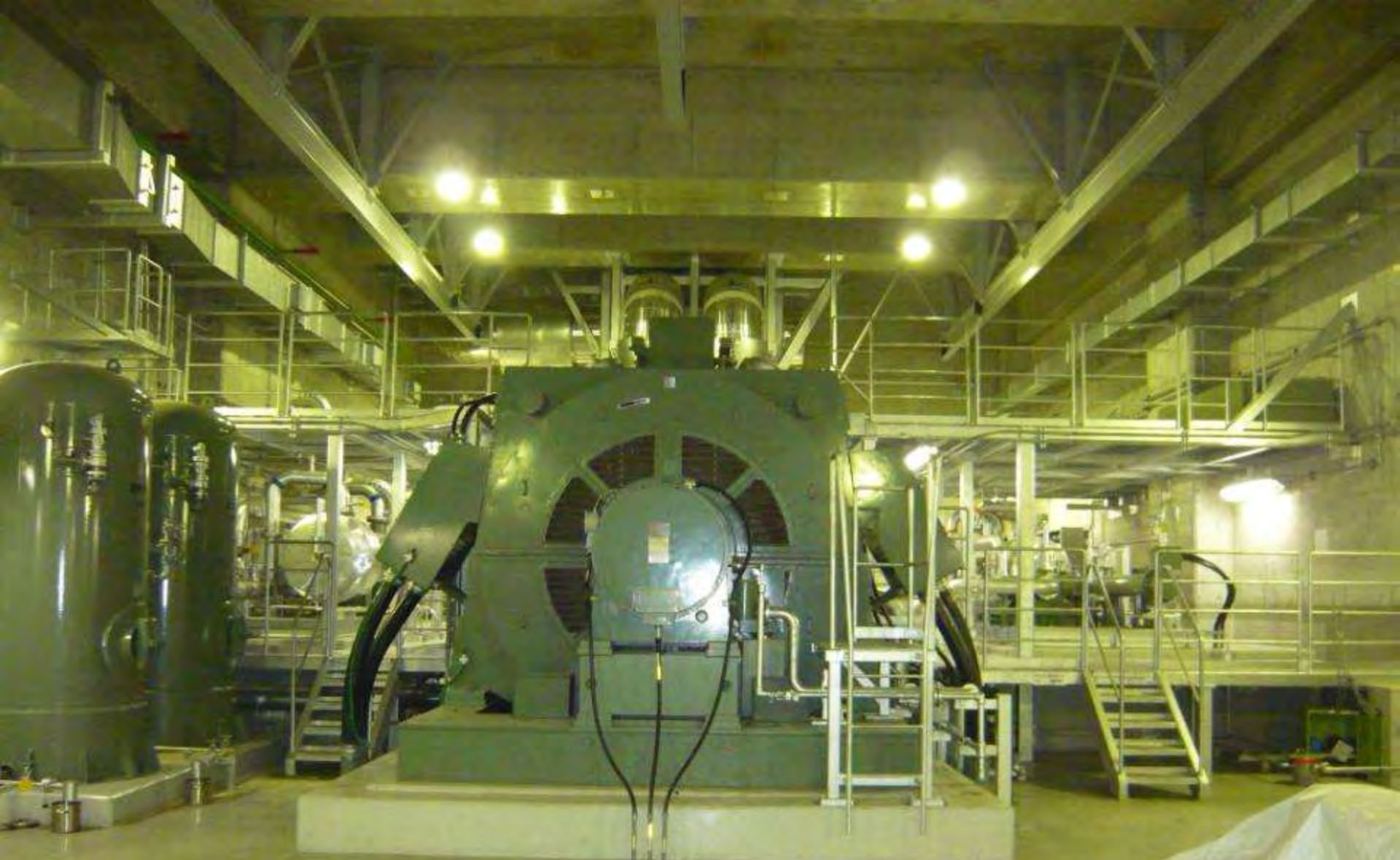
6号機空冷式非常用ディーゼル発電機
