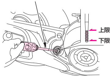
オイルレベルゲージ
