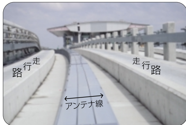
アンテナ線敷設 走行路の間に、3対のアンテナ線が敷設されています。
